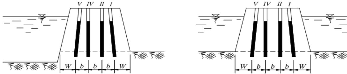
a) Sơ đồ chịu áp lực nước một phía
