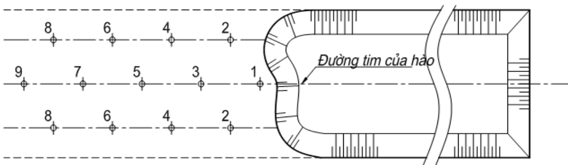
Hình 2 - Sơ đồ trình tự đốt dây cháy chậm khi nổ mìn để đào tuyến hào hẹp
