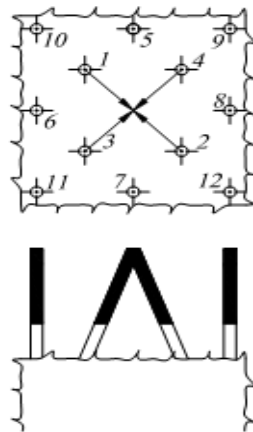
Hình 7 - Sơ đồ nổ mìn toàn bộ các lỗ khoan nhỏ
