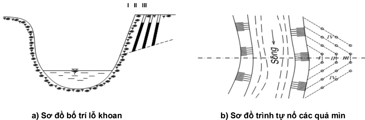
Hình 11 - Sơ đồ bố trí nổ mìn lỗ sâu để đắp vào công trình mới
