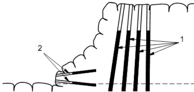
Hình 4 - Nổ phối hợp giữa các quả mìn trong lỗ khoan sâu và lỗ khoan nông
