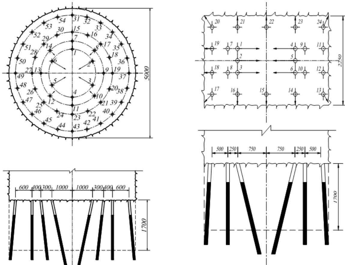
a) Công trình đào có mặt cắt hình tròn
