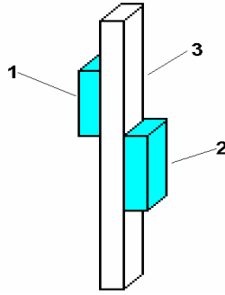
Hình 3 - Sơ đồ bố trí nổ mìn cắt các vật thể dài
